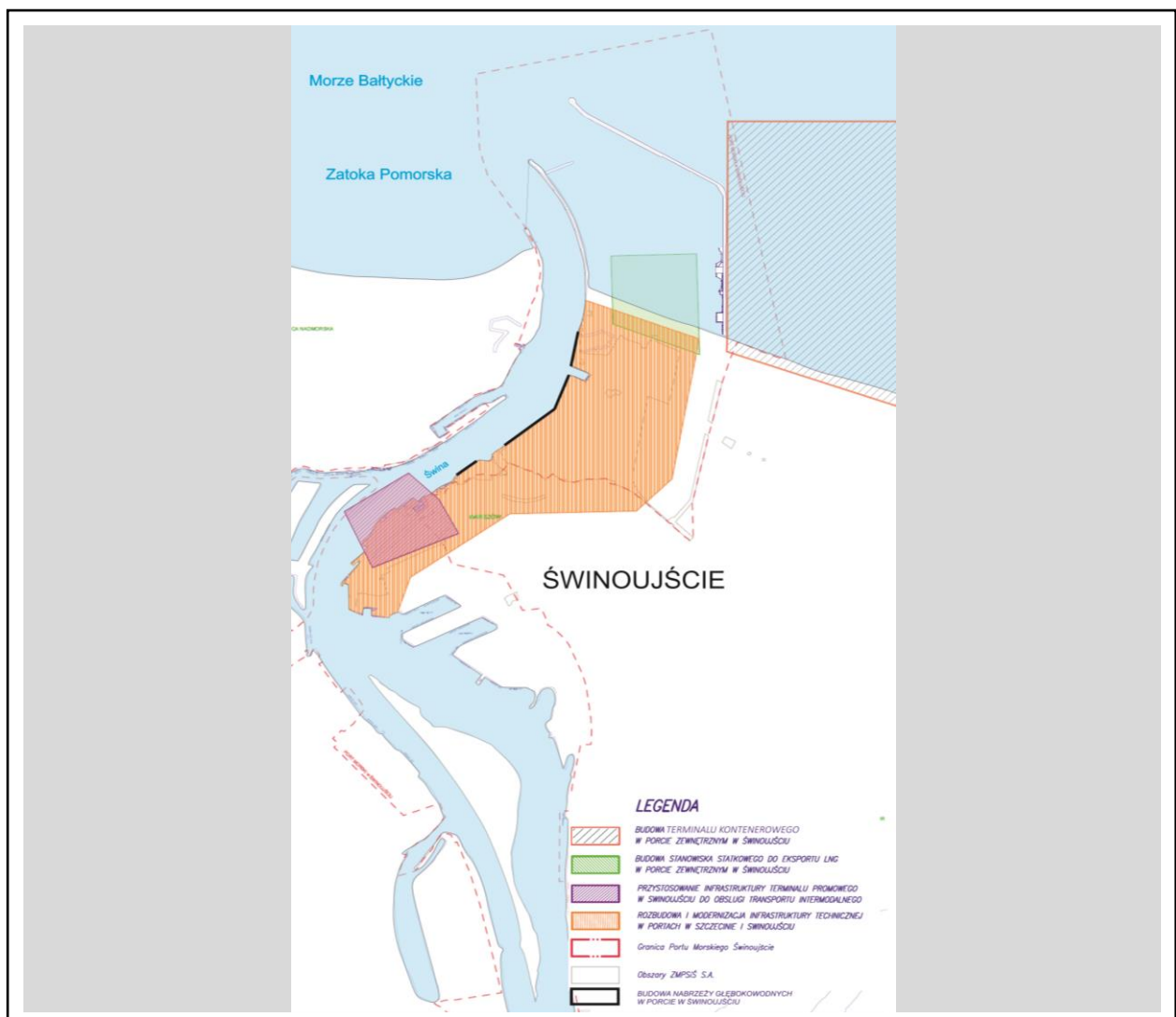
Rysunek 32 Projekty inwestycyjne w porcie morskim Świnoujście 68
