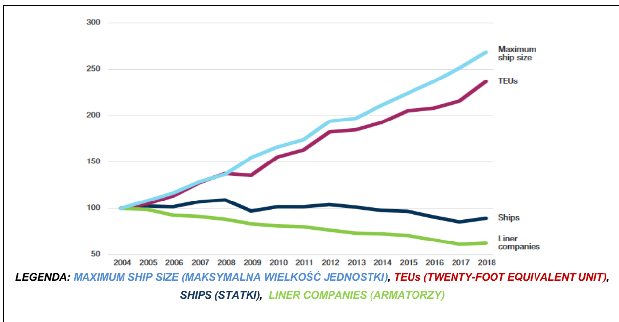
Rysunek 25 Kontenerowce oddawane do eksploatacji w latach 2004-2018 (rok bazowy 2004 = 100,00 %)
