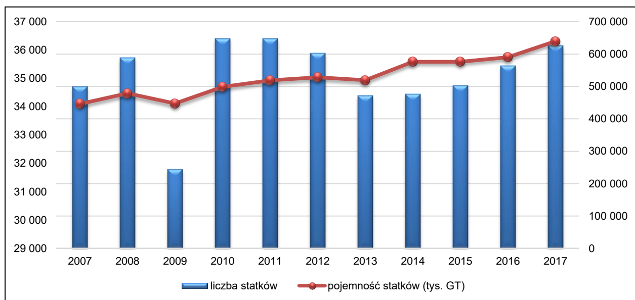
Rysunek 20 Dynamika obsługi statków w badanych portach: liczba statków łącznie (oś lewa; wykres słupkowy w kolorze niebieskim), łączna pojemność statków (tys. GT; oś prawa; wykres liniowy w kolorze czerwonym)
