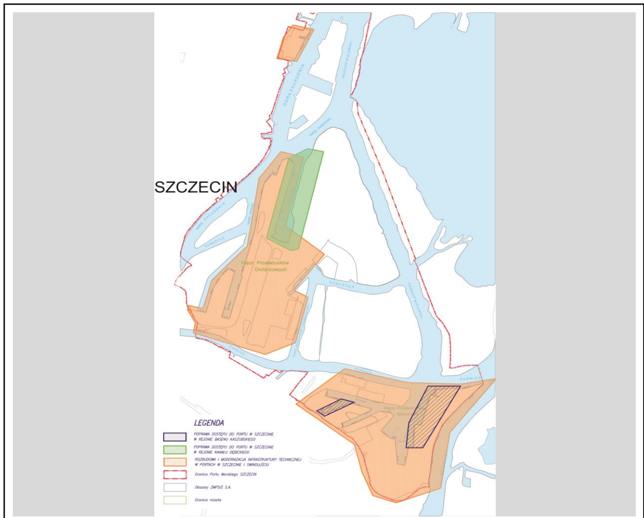
Rysunek 31 Projekty inwestycyjne w porcie morskim Szczecin
